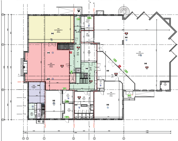
PO0 - begane grond nieuw 1:100
