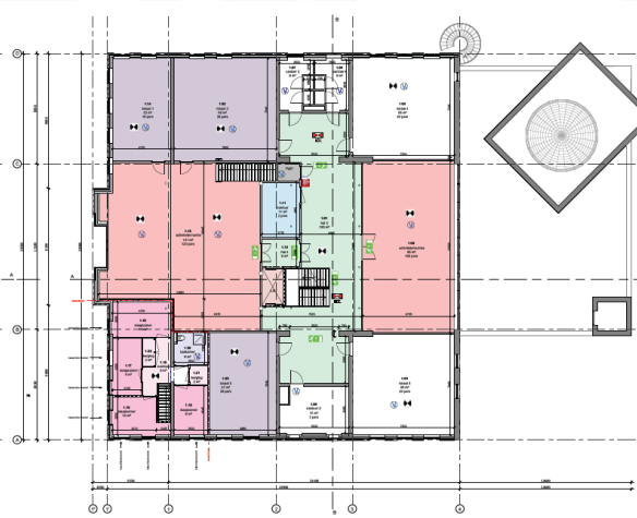
PO1 - eerste verdieping nieuw 1:100
